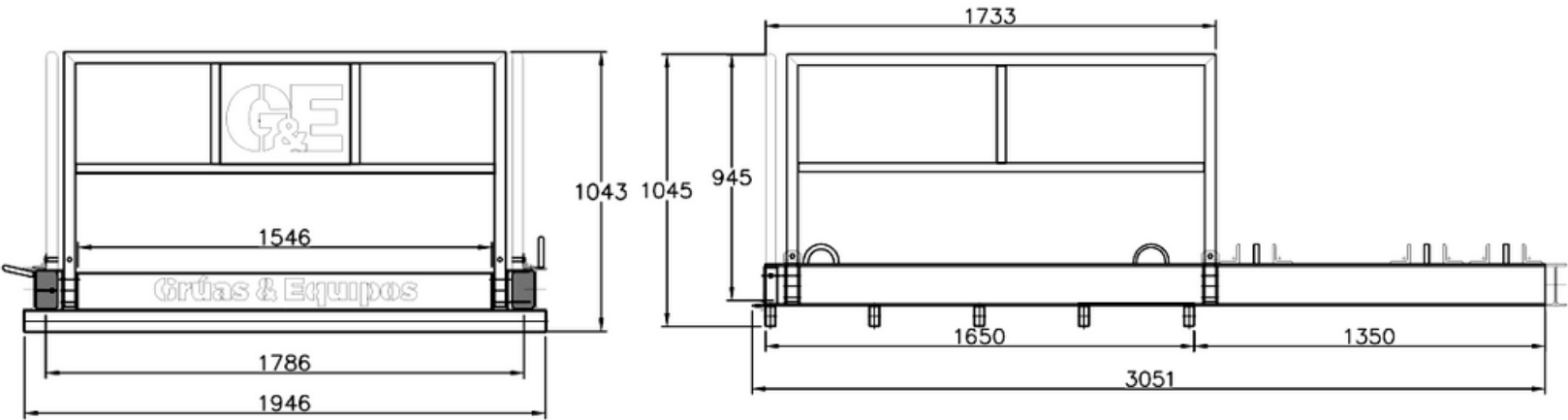
VISTA LATERAL
